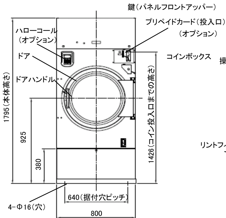
正面図
