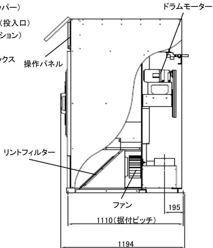
側面図
