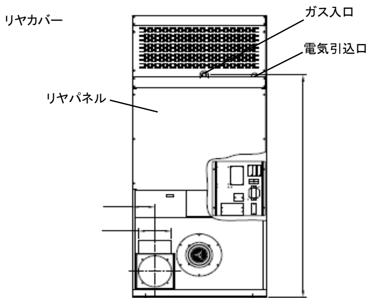
背面図
